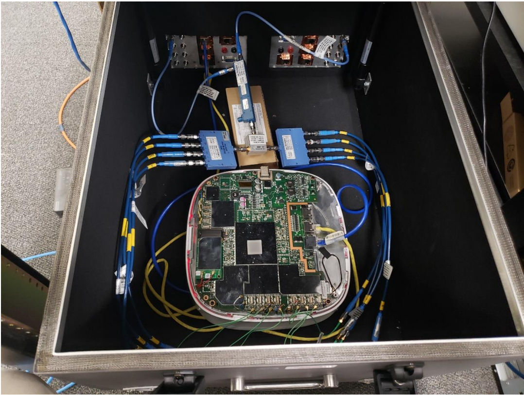
EUT Photo
