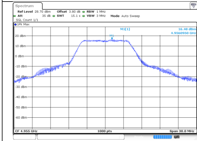
4950-10MHz-802.11a-1-a
