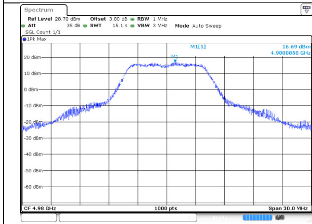
4980-10MHz-802.11a-1-a
