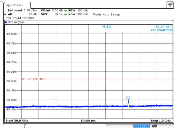
4950-10MHz-802.11n-1-a
