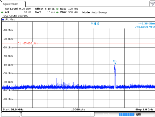
4950-10MHz-802.11a-2-a
