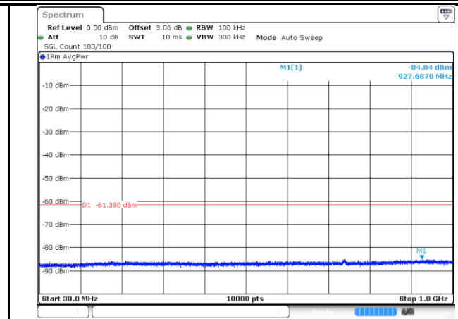
4950-10MHz-802.11n-2-b
