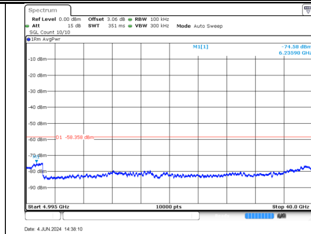
4950-20MHz-802.11n-2-b
