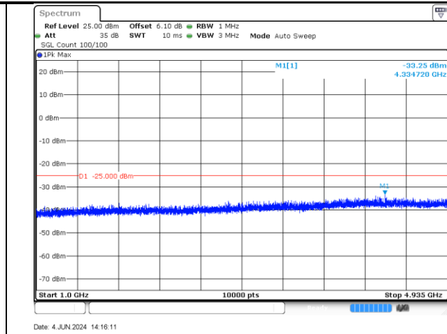
4955-10MHz-802.11a-2-a
