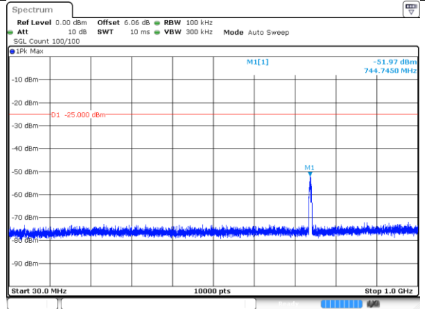
4950-10MHz-802.11a-2-a
