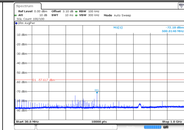
4950-20MHz-802.11n-2-a
