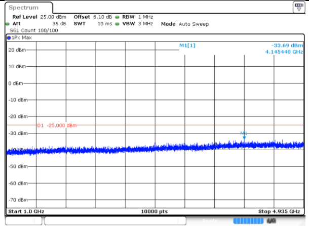
4950-10MHz-802.11a-2-a
