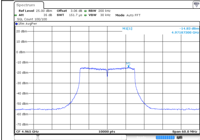
4965-20MHz-802.11n-1-a
