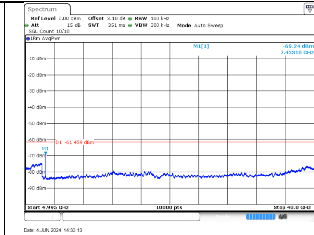
4955-10MHz-802.11n-2-a
