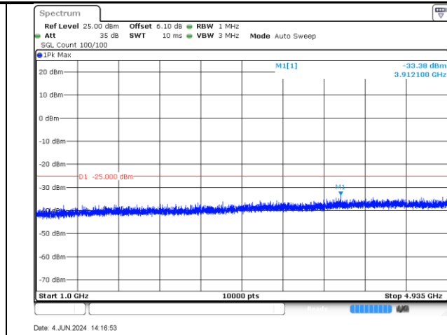
4980-10MHz-802.11a-2-a
