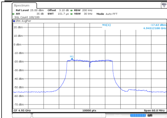
4950-20MHz-802.11n-2-a
