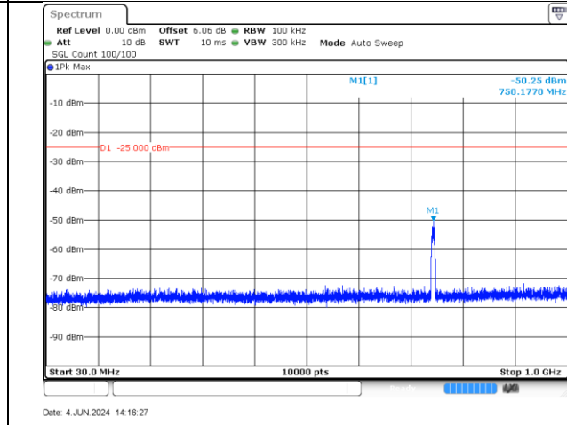
4955-10MHz-802.11a-2-b
