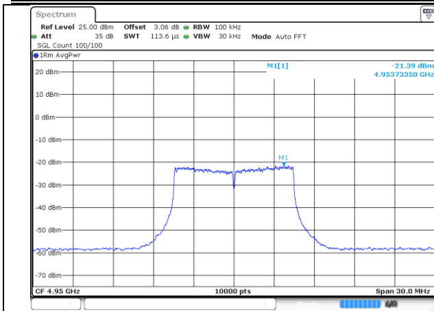
4950-10MHz-802.11n-2-b
