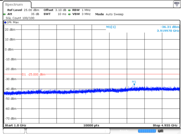
4955-10MHz-802.11a-1-a
