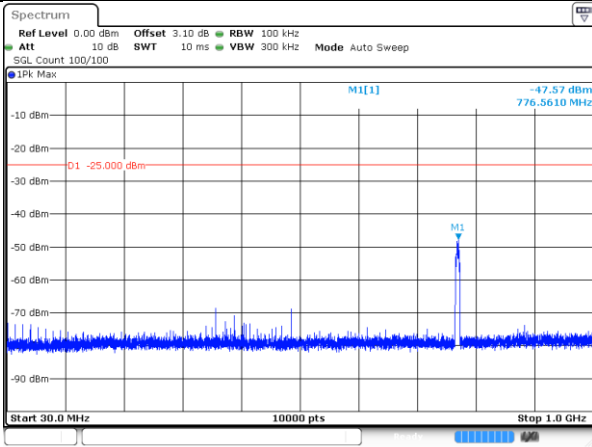
4980-10MHz-802.11a-1-a
