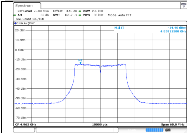
4965-20MHz-802.11n-1-a
