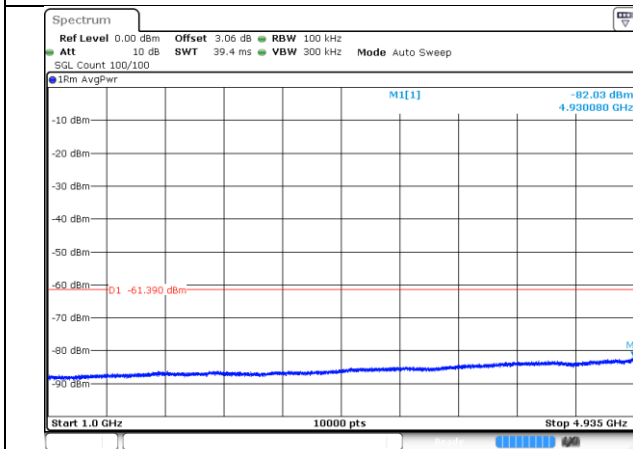
4950-10MHz-802.11n-2-b
