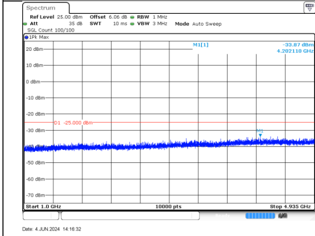
4955-10MHz-802.11a-2-b
