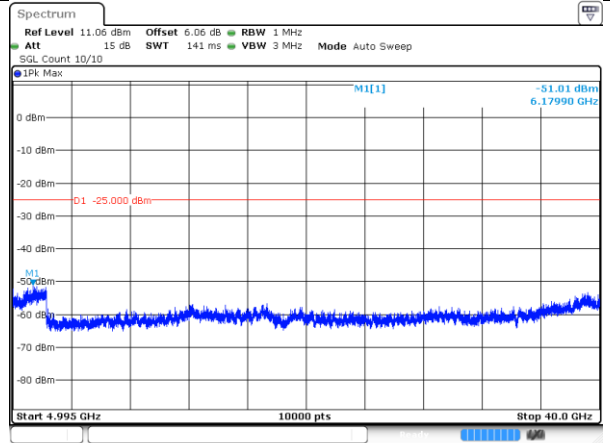
4950-10MHz-802.11a-2-b
