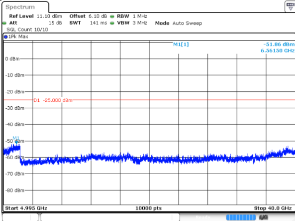
4950-10MHz-802.11a-2-a
