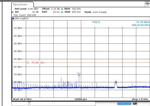
4965-20MHz-802.11n-1-a
