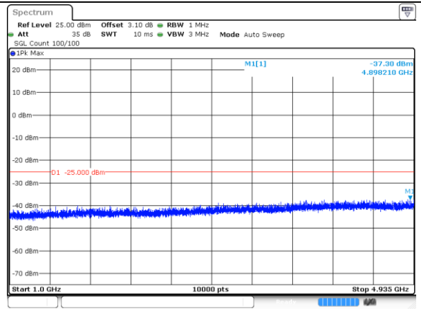
4950-10MHz-802.11a-1-a
