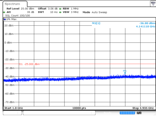
4950-10MHz-802.11a-1-a
