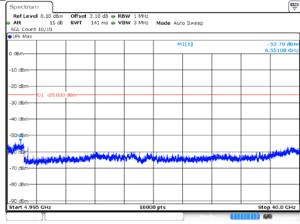
4950-10MHz-802.11a-1-a
