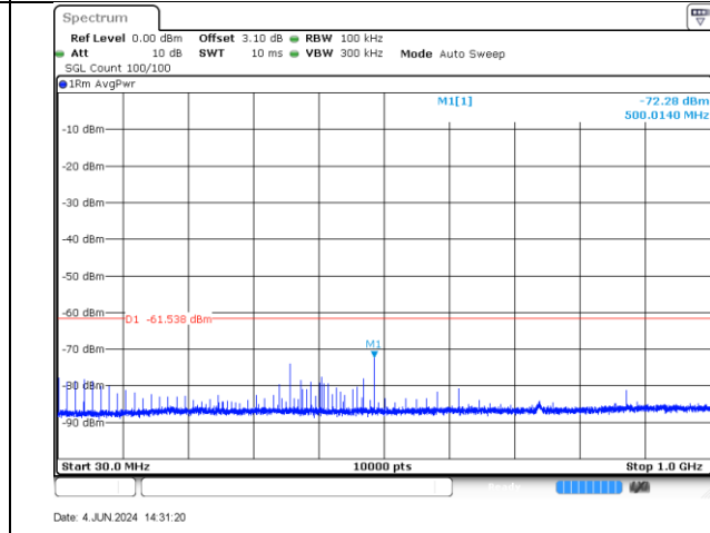
4950-10MHz-802.11n-2-a
