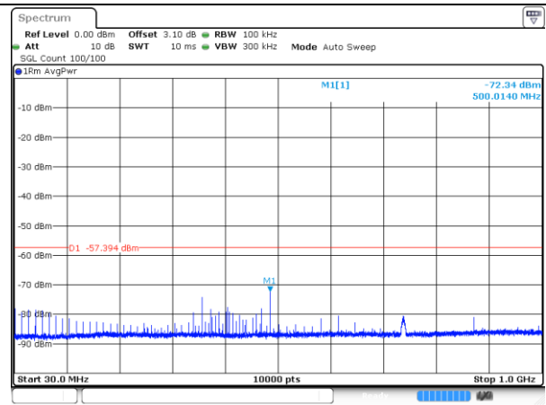
4950-10MHz-802.11n-1-a
