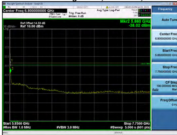
Antenna A
