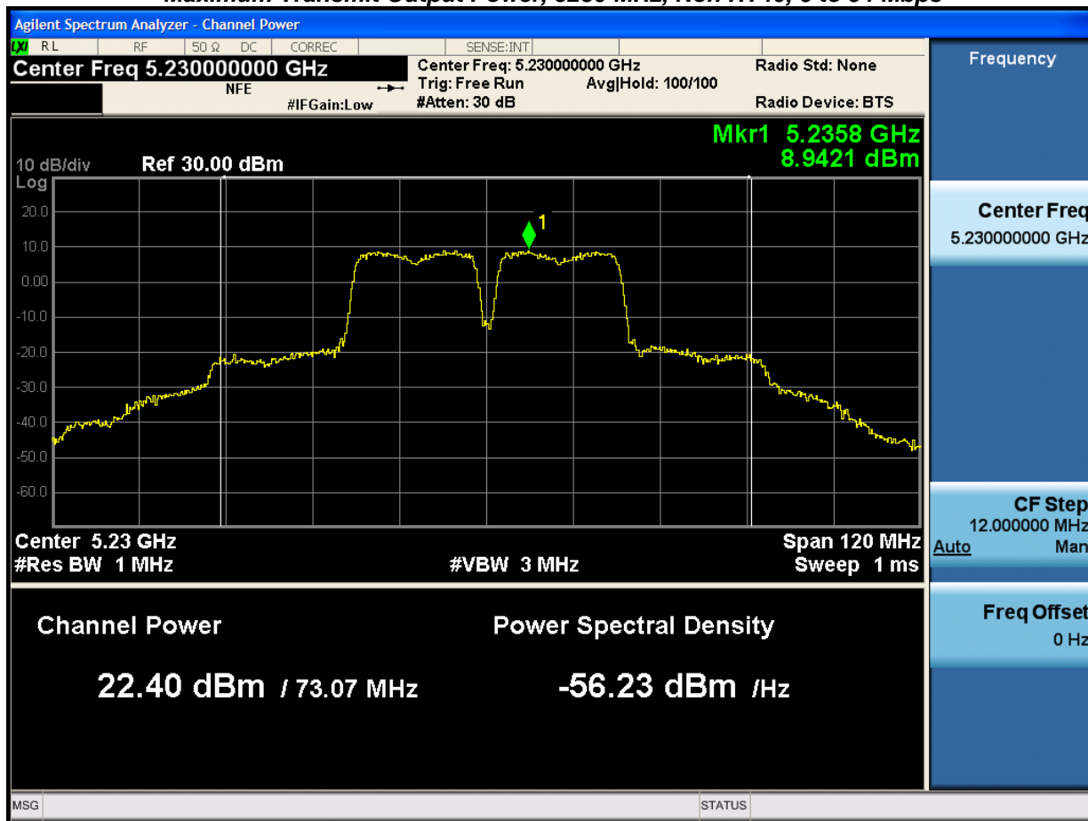
Antenna A
