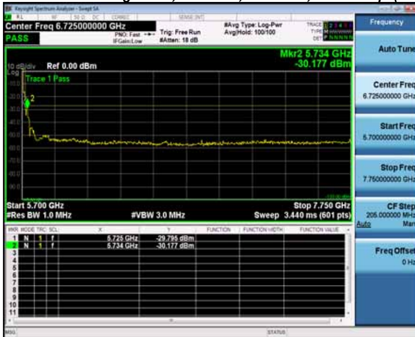
Antenna A
