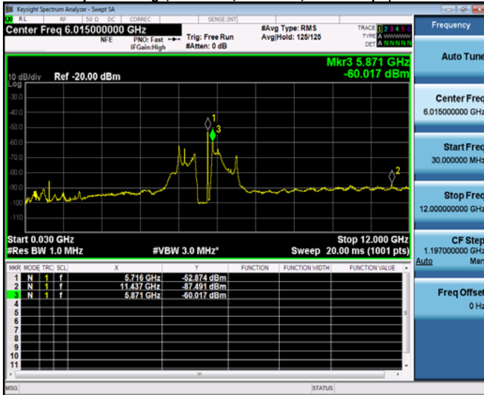
Antenna A
