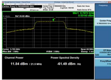
Antenna A
