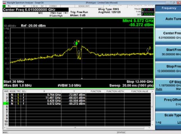
Antenna A
