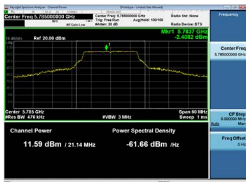
Antenna A
