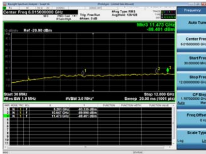
Antenna A
