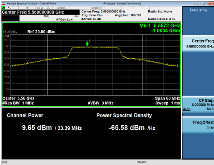
Antenna A
