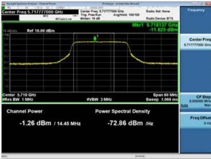
Antenna A
