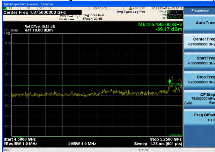
Antenna A
