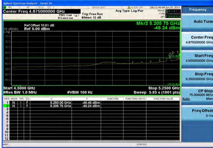
Antenna A
