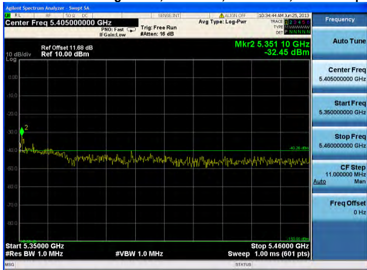
Antenna A
