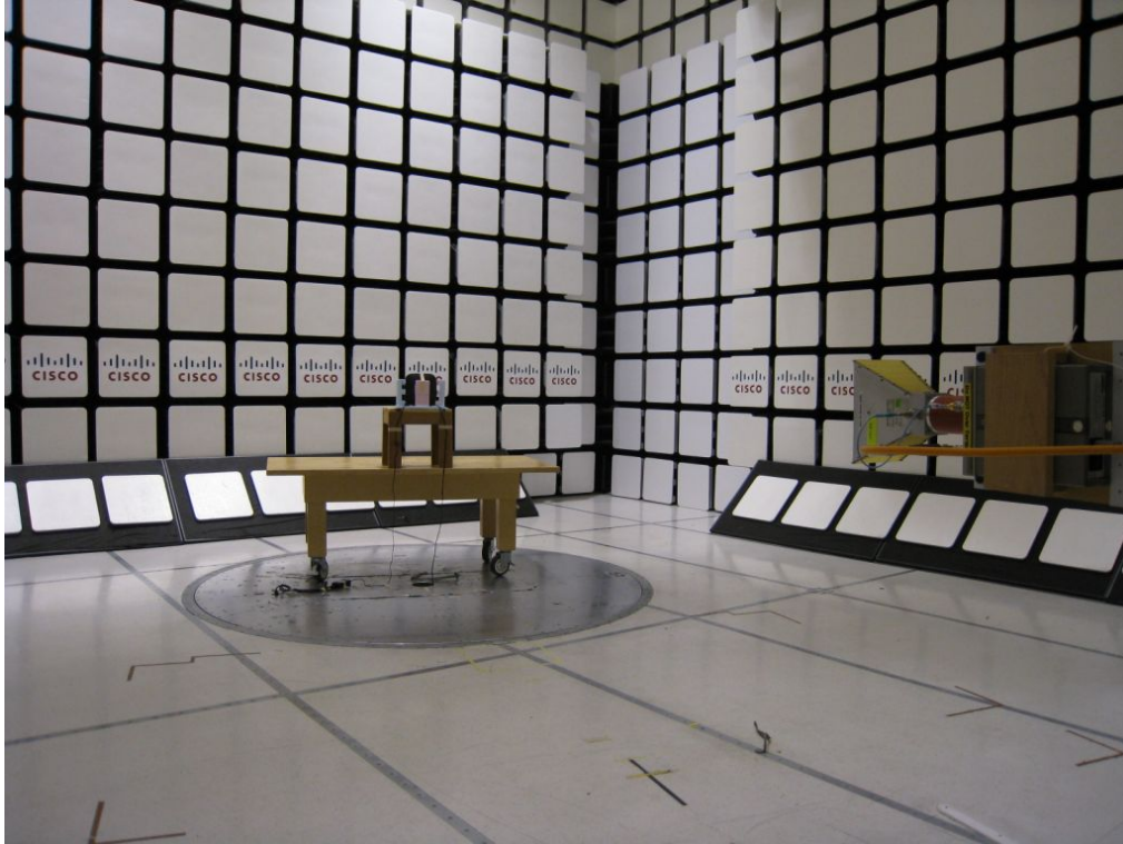
1-18GHz Test Setup
