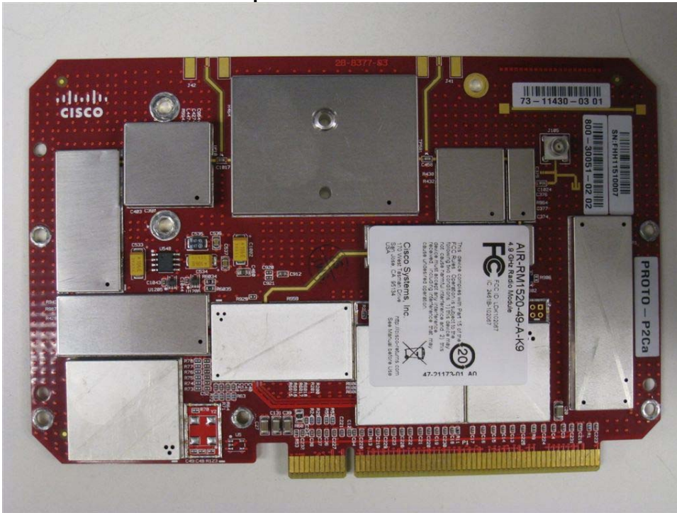
AIR-RM1520-49 Bottom
