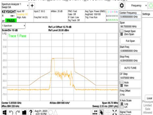
802.11ax_20MHz_Chain1_5955MHz_RU26_0
