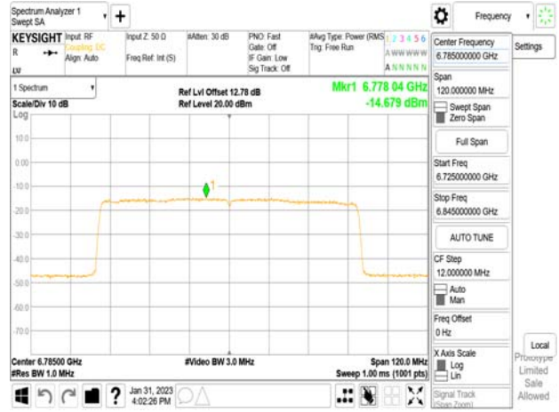
802.11ax_80MHz_Chain1_6785MHz_RU484_66
