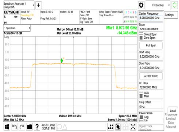
802.11ax_80MHz_Chain1_5985MHz_RU484_65
