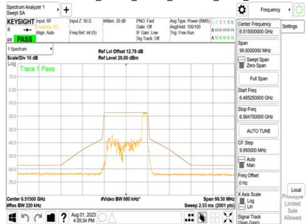
802.11ax_20MHz_Chain0_6515MHz_RU52_40
