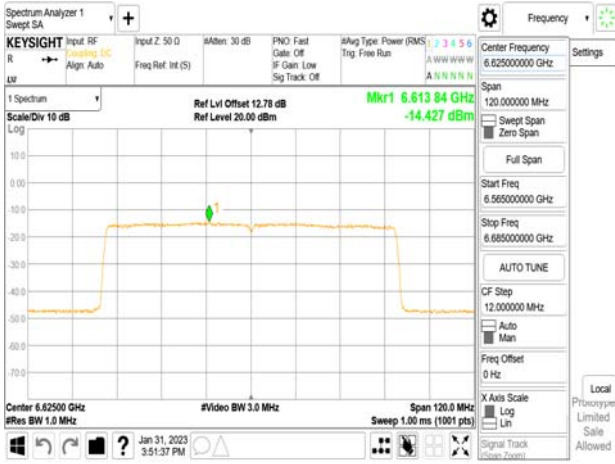
802.11ax_80MHz_Chain1_6625MHz_RU484_65
