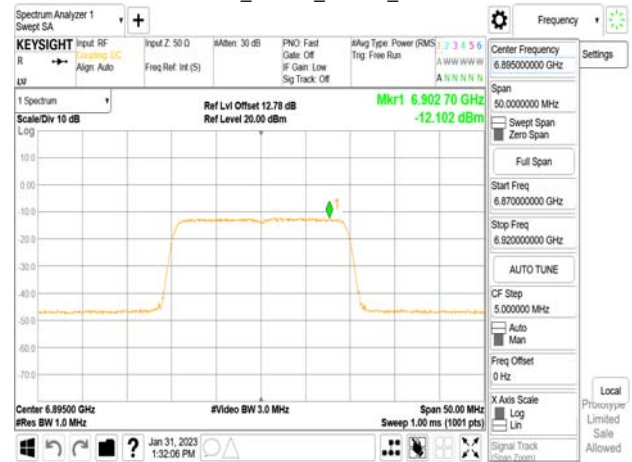
802.11ax_20MHz_Chain1_6895MHz
