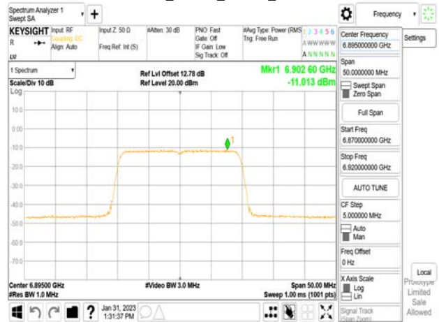
802.11ax_20MHz_Chain0_6895MHz_RU26_0
