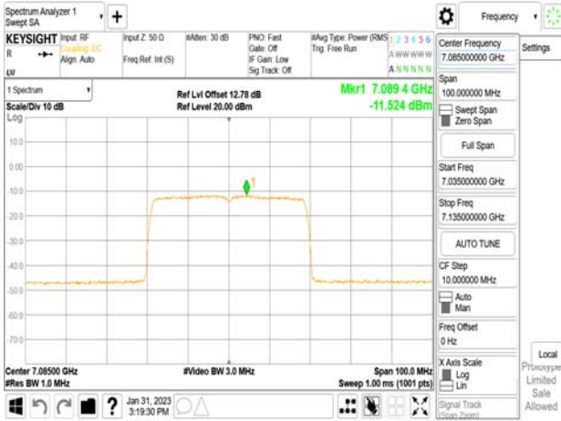
802.11ax_40MHz_Chain1_7085MHz_RU242_62
