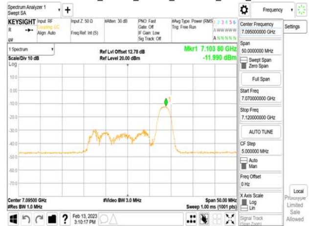
802.11ax_20MHz_Chain1_7095MHz_RU26_8
