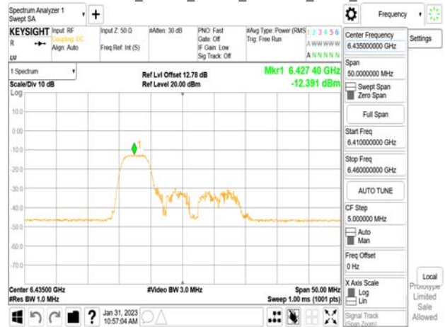
802.11ax_20MHz_Chain0_6435MHz_RU52_37
