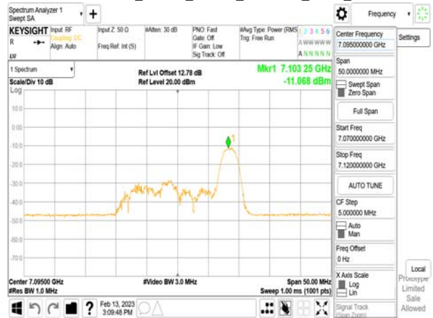
802.11ax_20MHz_Chain0_7095MHz_RU52_40
