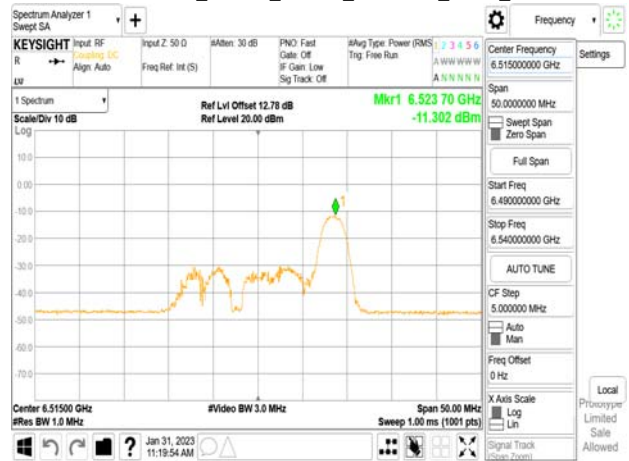
802.11ax_20MHz_Chain1_6515MHz_RU52_40
