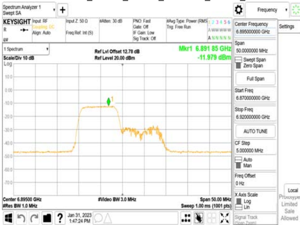
802.11ax_20MHz_Chain1_6895MHz_RU106_53
