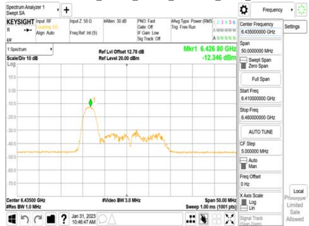
802.11ax_20MHz_Chain0_6435MHz_RU52_37
