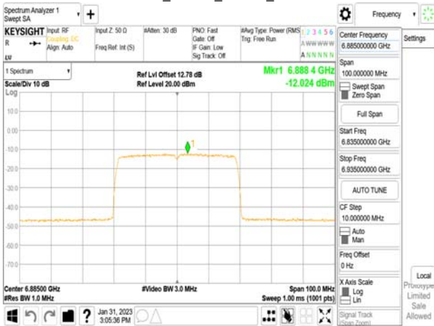
802.11ax_40MHz_Chain1_6885MHz
