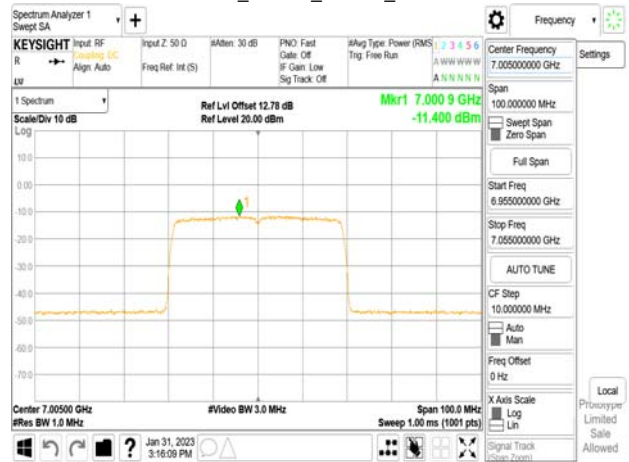
802.11ax_40MHz_Chain1_7005MHz
