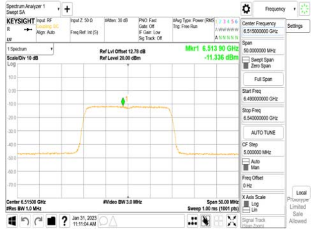
802.11ax_20MHz_Chain1_6515MHz_RU26_8
