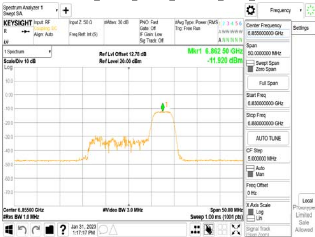
802.11ax_20MHz_Chain1_6855MHz_RU52_40
