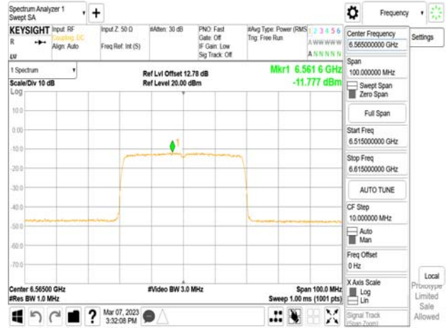
802.11ax_40MHz_Chain1_6565MHz_RU242_61
