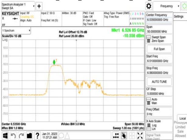
802.11ax_20MHz_Chain0_6535MHz_RU52_37
