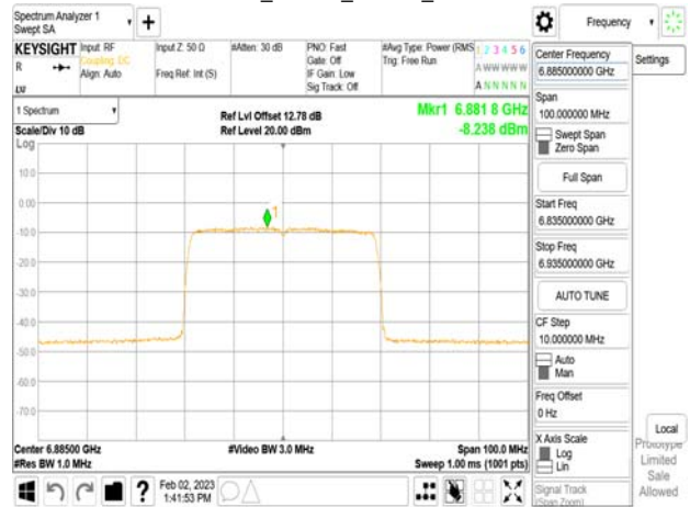
802.11ax_40MHz_Chain0_6885MHz
