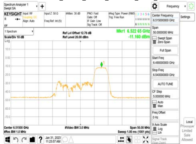
802.11ax_20MHz_Chain1_6515MHz_RU52_40
