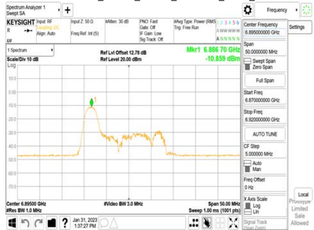
802.11ax_20MHz_Chain0_6895MHz_RU26_0
