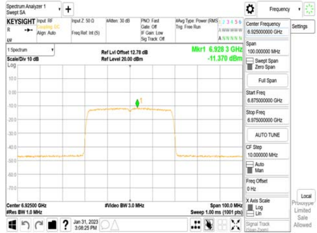
802.11ax_40MHz_Chain1_6925MHz_RU242_61
