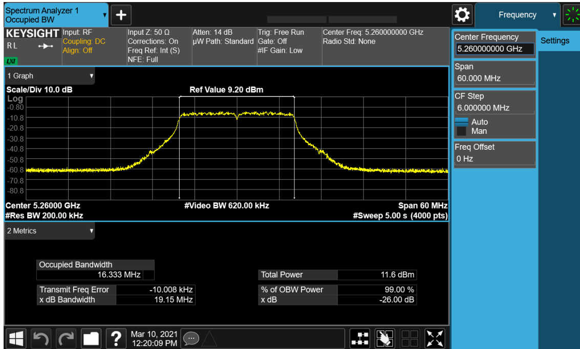
Antenna A
