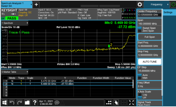
Antenna A
