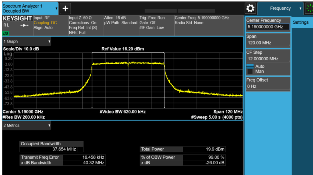
Antenna A
