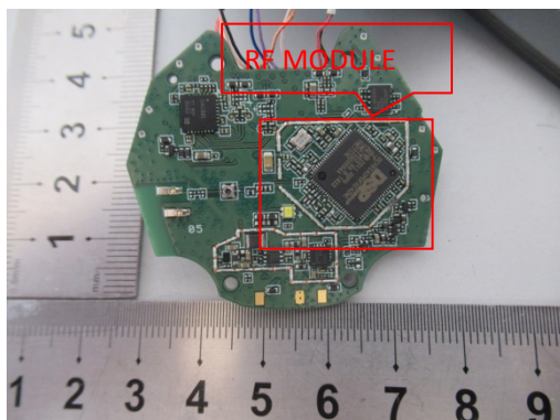
CP-HS-WL-562-N-US -PCB 2
