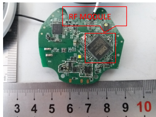
CP-HS-WL-561-N-US -PCB
