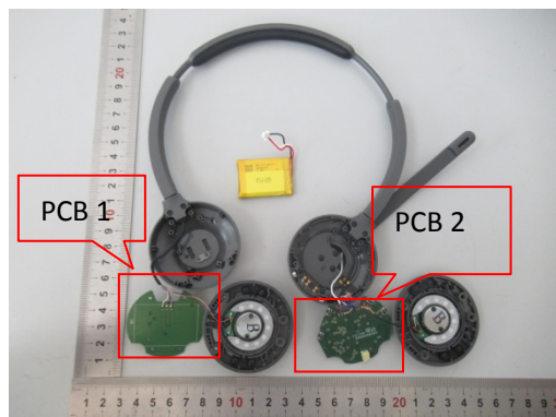
CP-HS-WL-562-N-US -PCB 2
