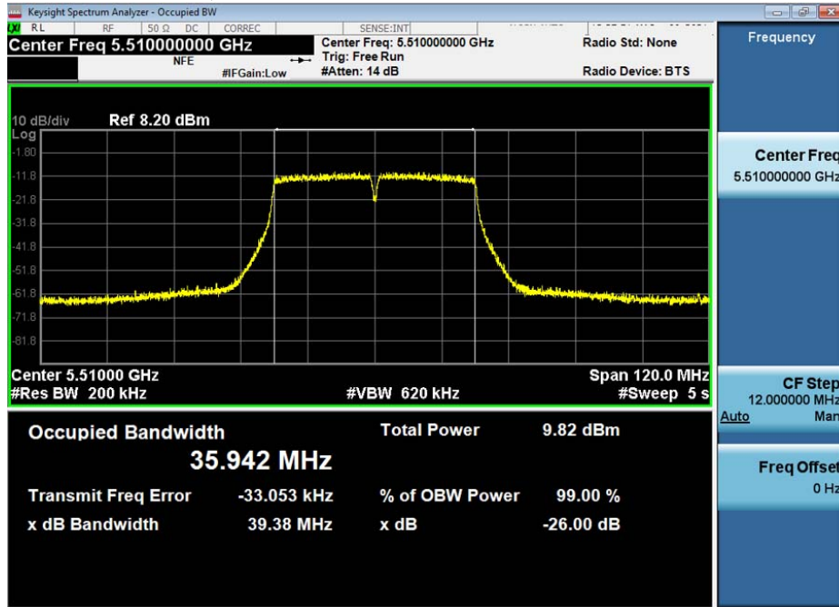
Antenna A
