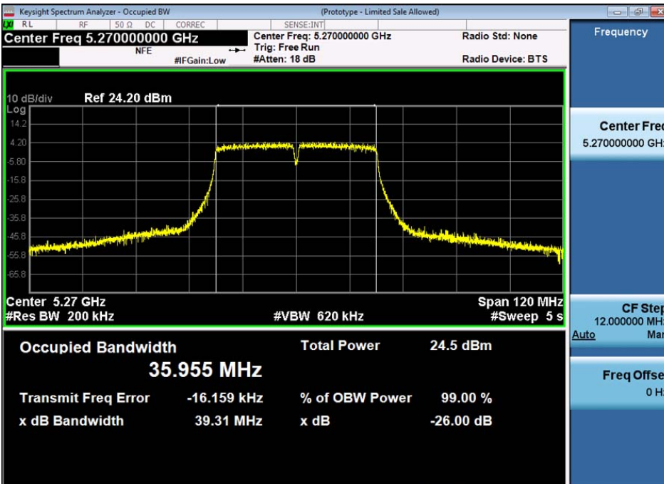
Antenna A
