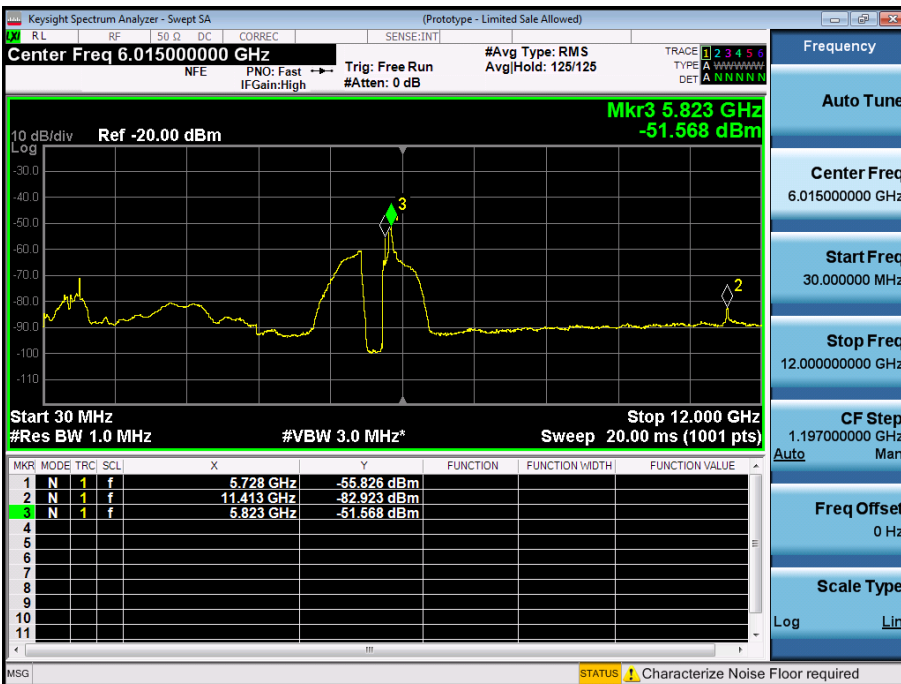
Antenna A
