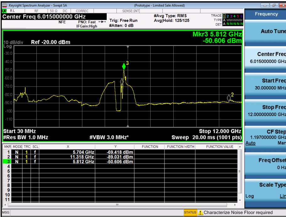
Antenna A
