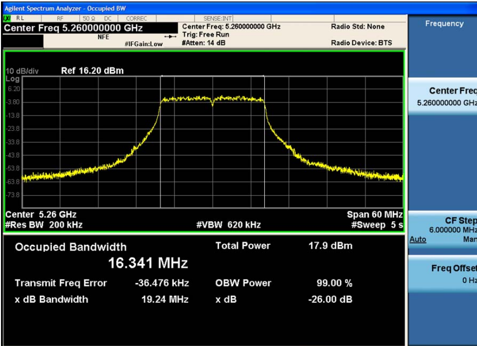
Antenna A
