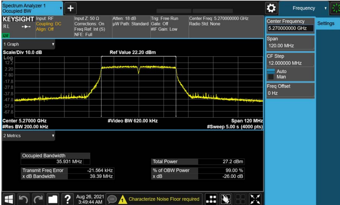
Antenna A
