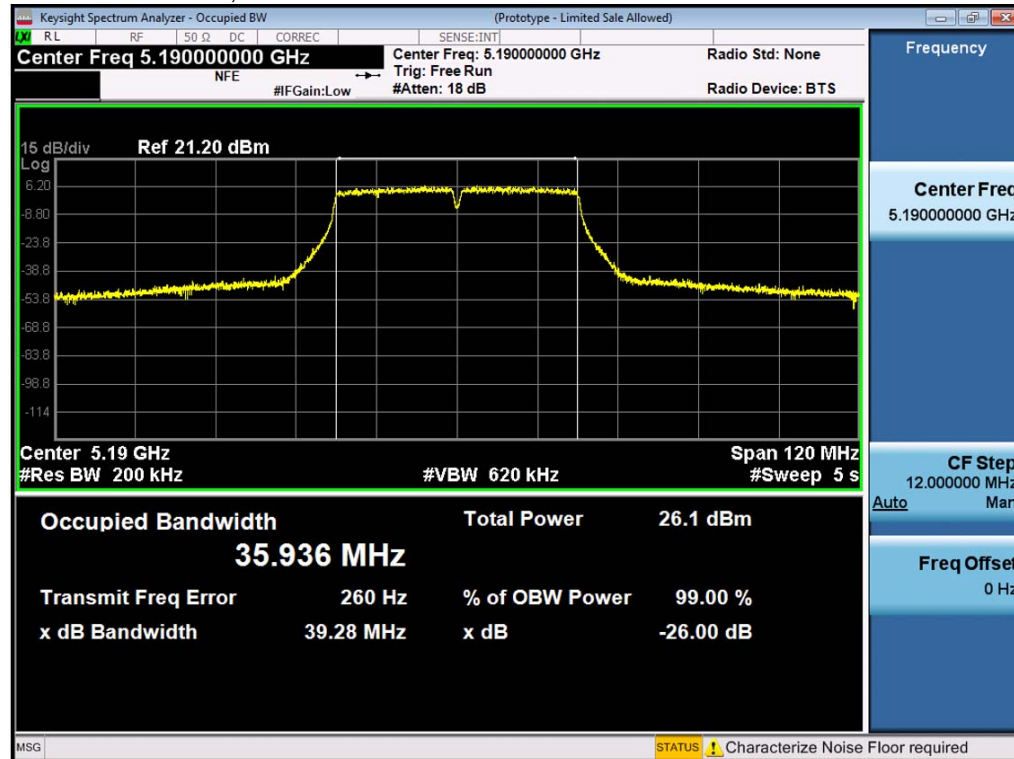
Antenna A
