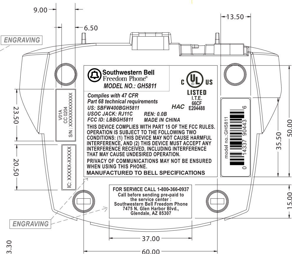
GH5811 BASE
