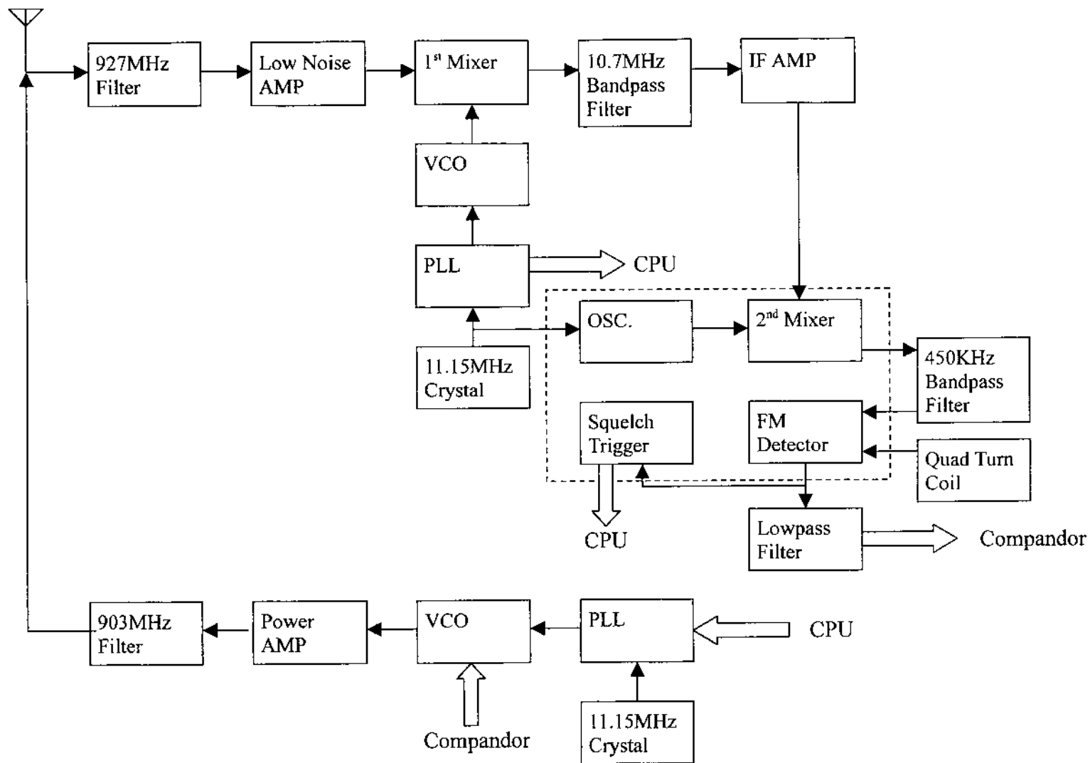
FF2150 900MHz phone base RF module block diagram
