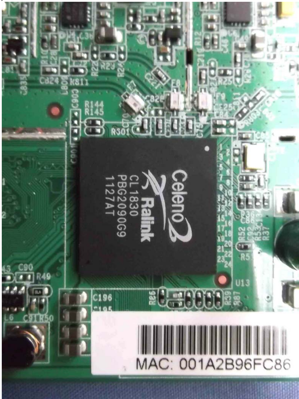
(12) EUT Photo
