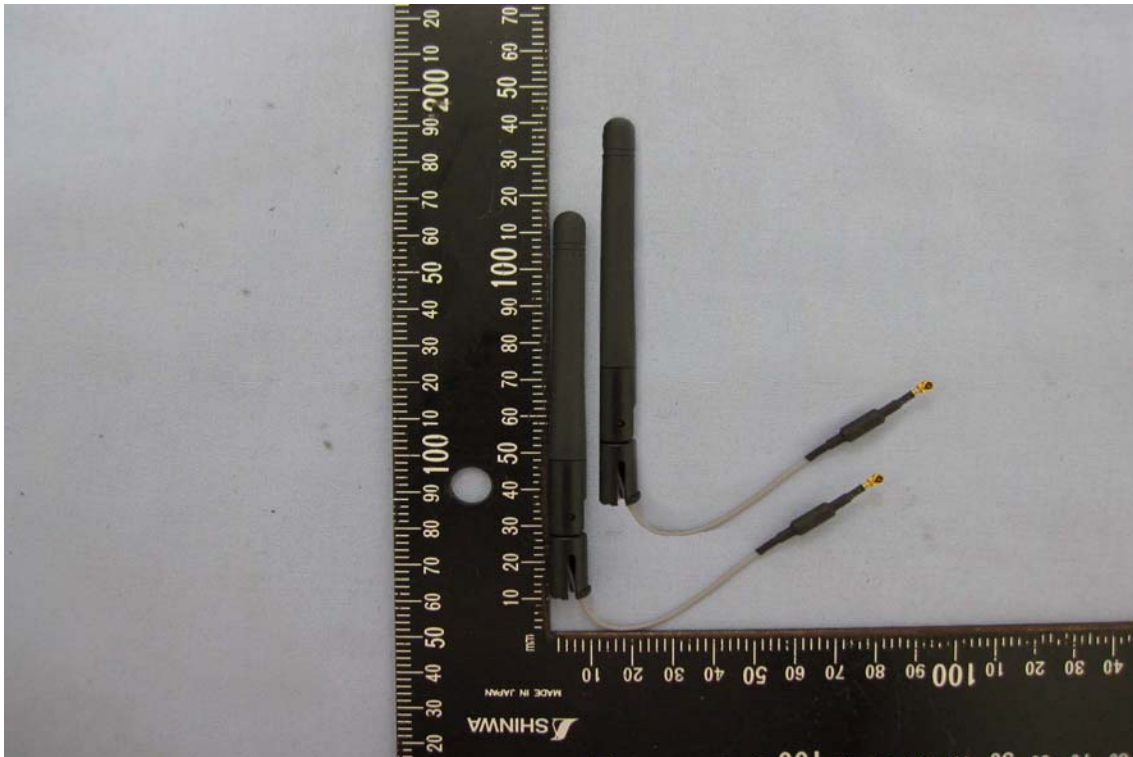
Dipole Antenna / 6602113051-090
