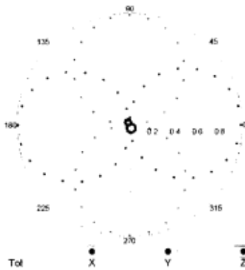
f=600 MHz, TEM, 0^\circ
