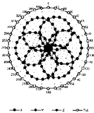
f = 600 MHz, TEM 111110EXX
