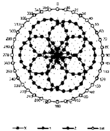
f = 500 MHz, TEM in110EXX
