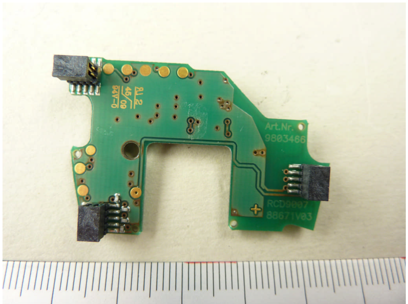
100886_2pcb1
