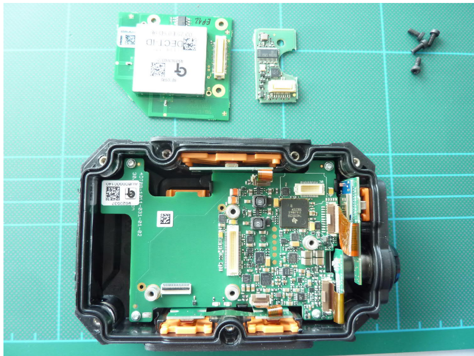
170685EUTinternal06: Inside view 4
