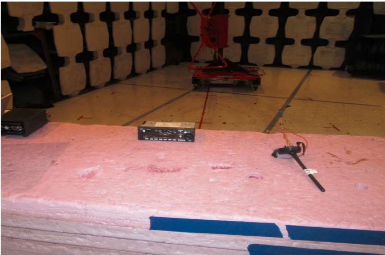
30-1000MHz
