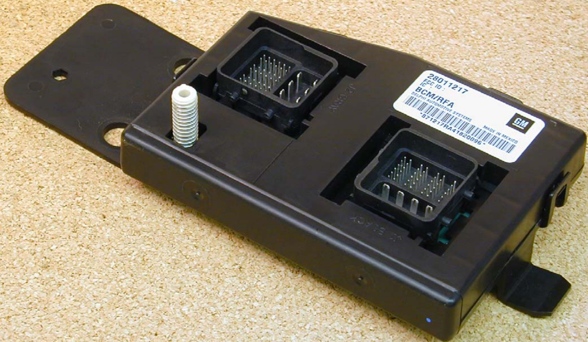
DUT (top)
