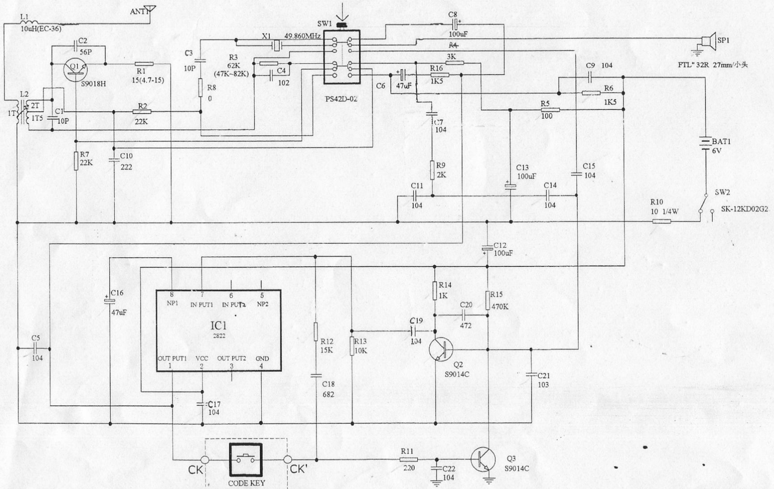
WT-A1.6-D(控制板) (铜箔镀镍,板厚1.6mm)
