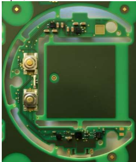
Bottom PCB
