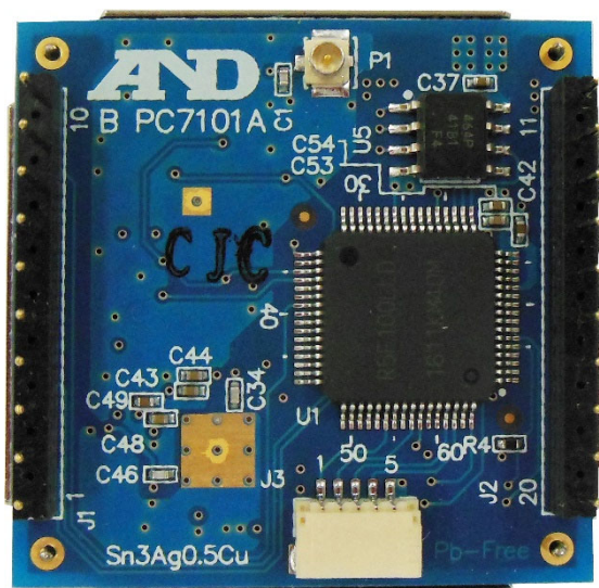
裏面 Bottom
