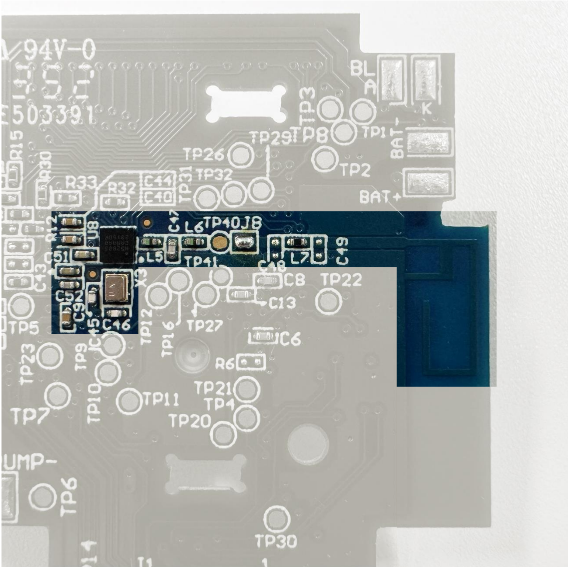
Bluetooth IC & PCB Antenna
