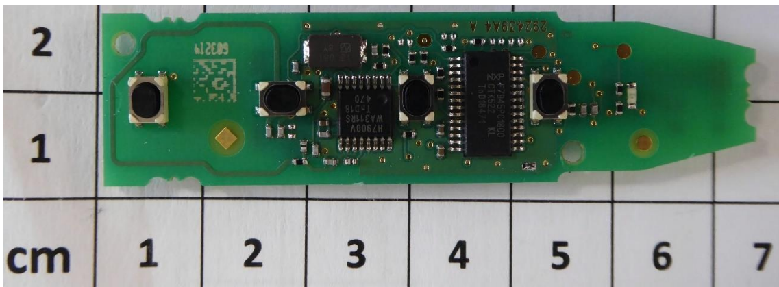
PCB bottom
