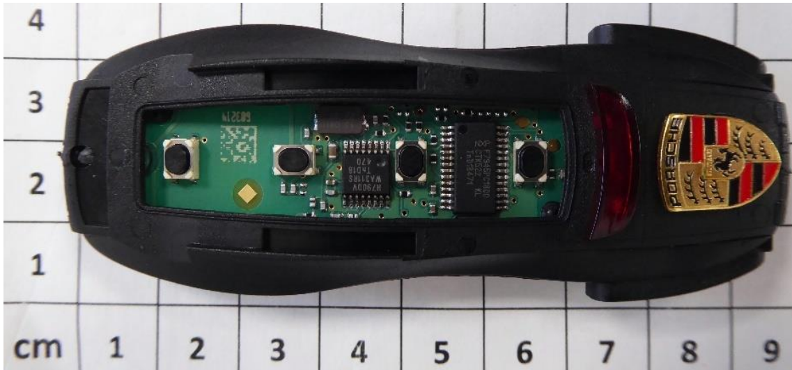
PCB bottom
