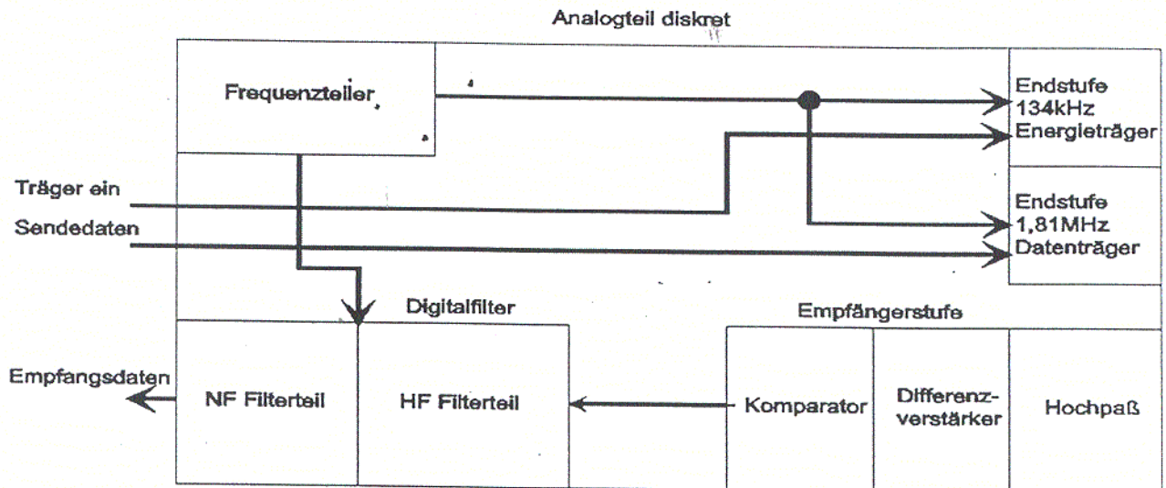
Abbildung 2 Detail Analogteil
