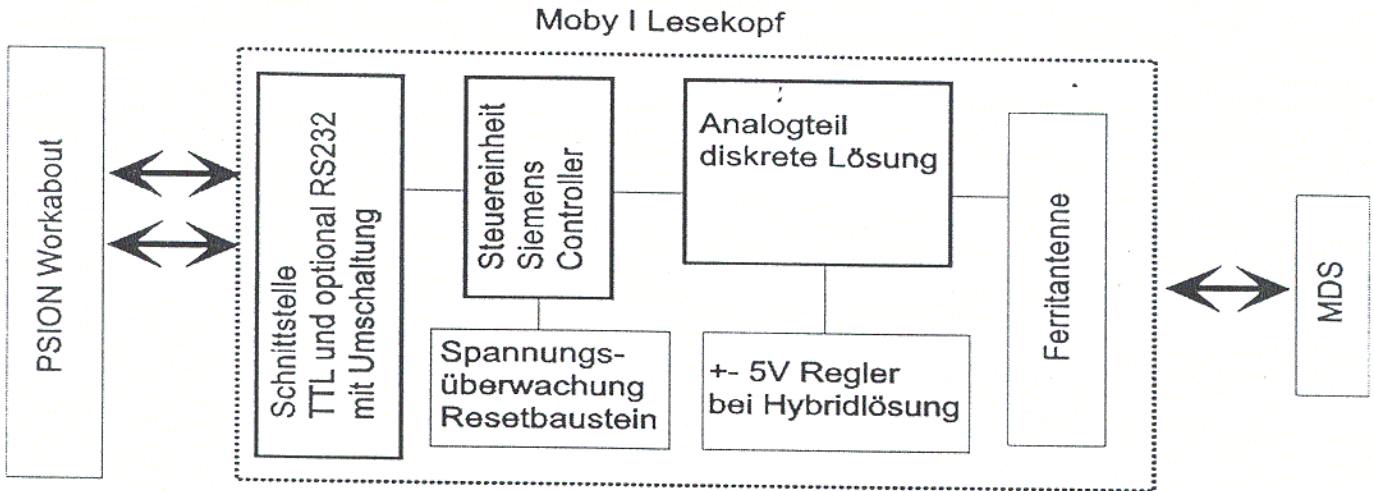
Abbildung 1 Blockschaltbild
