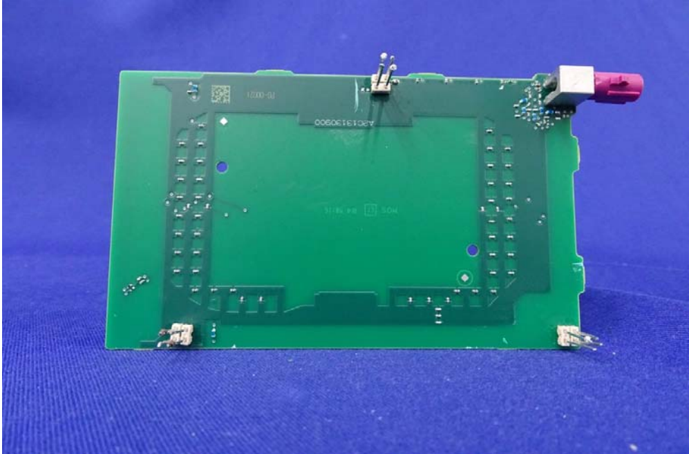
(8) EUT Photo
