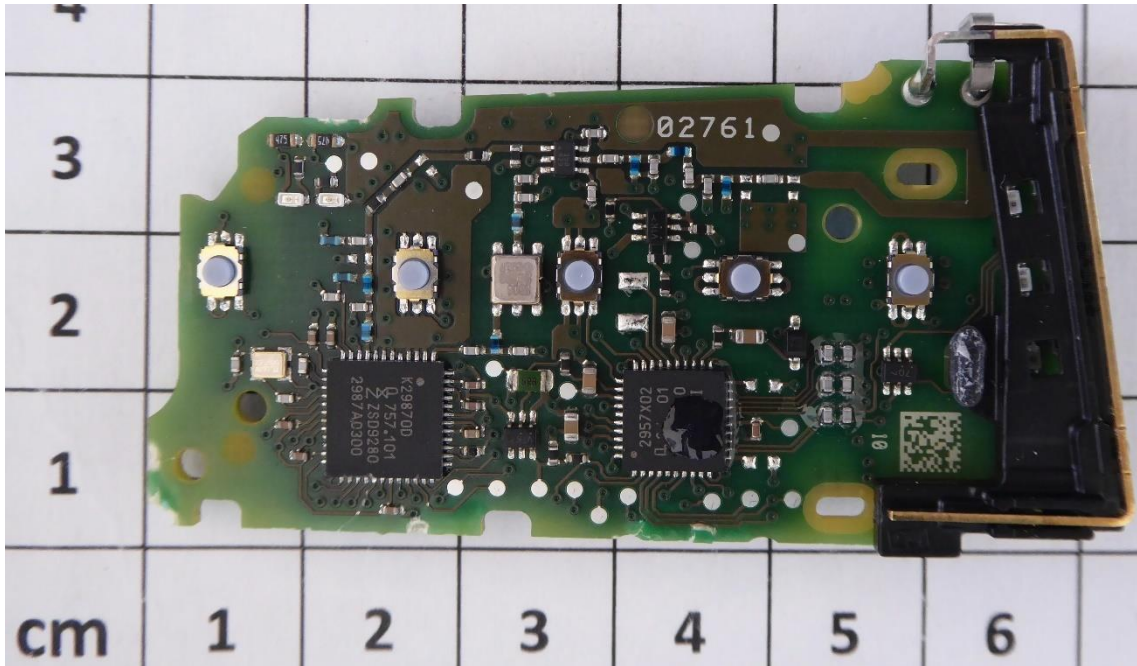
PCB top
