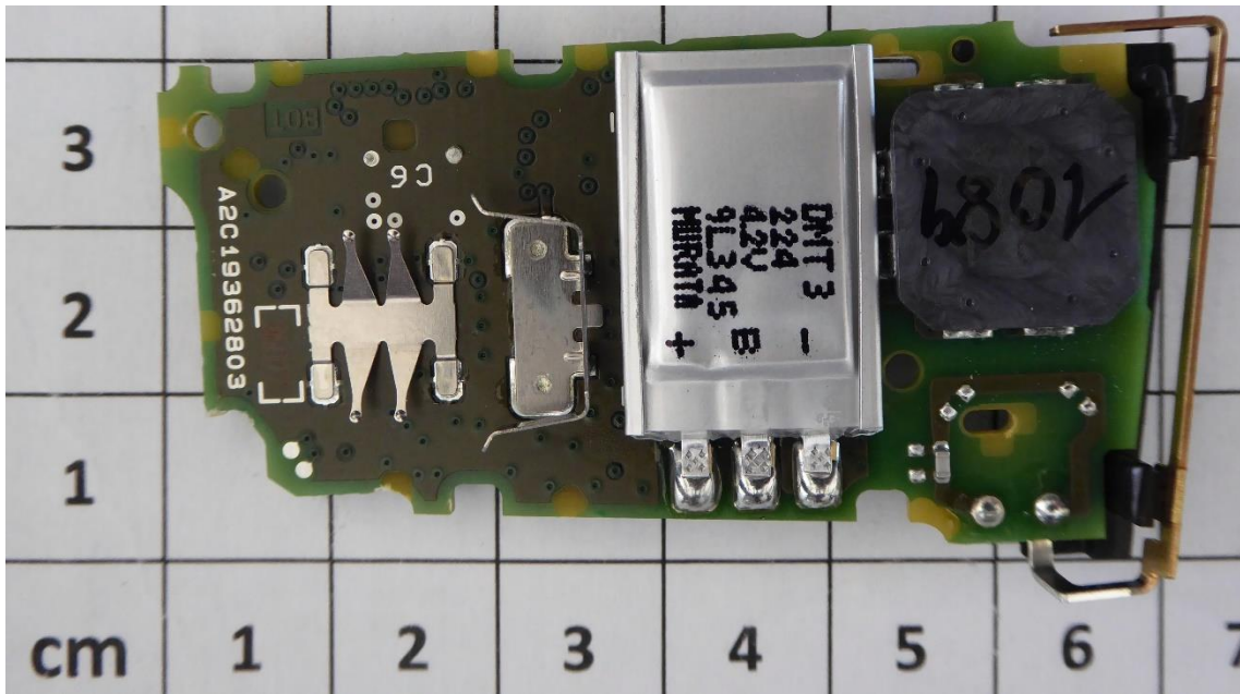
PCB bottom
