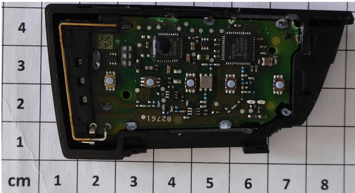
PCB top
