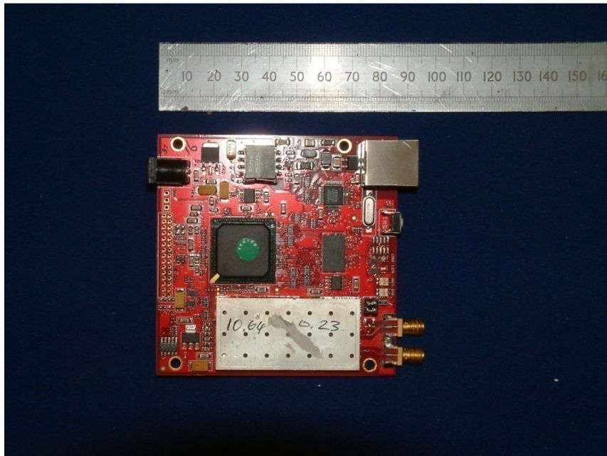
CPE Module S/N 4344 (Top Face)
