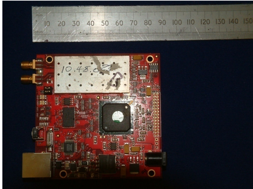
CPE Module S/N 4371 (Top Face)
