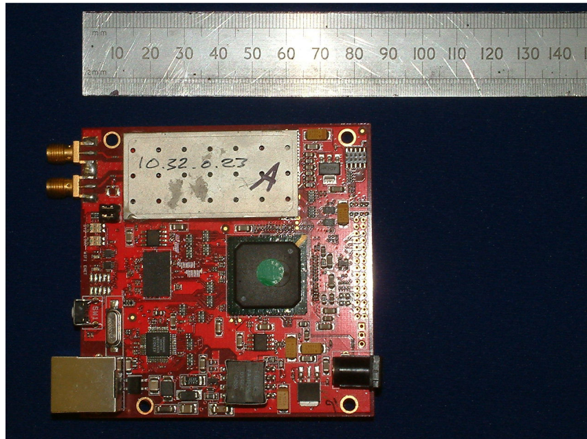
CPE Module S/N 4381 (Top Face)
