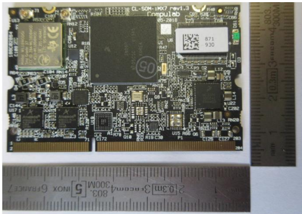
WLAN module
