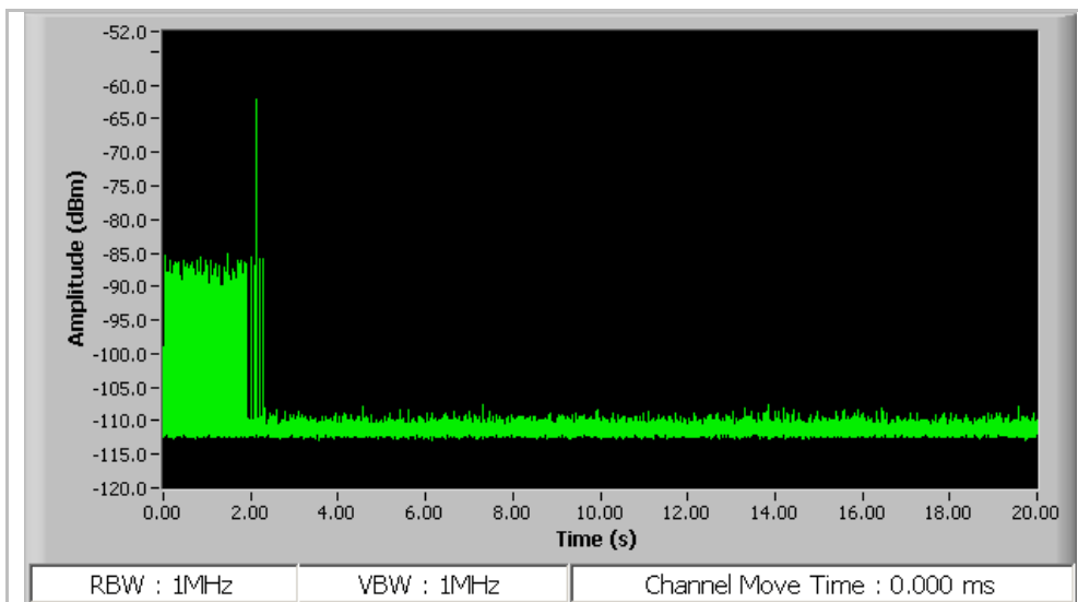
CH Move time - 802.11ac-80MHz-5290MHz
