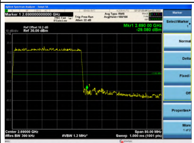
n41_40MHz_Upper Band Edge
