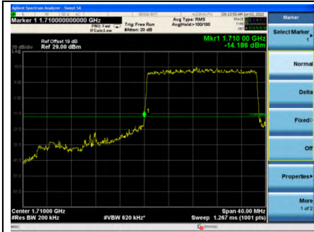
n66_20MHz_Lower Band Edge
