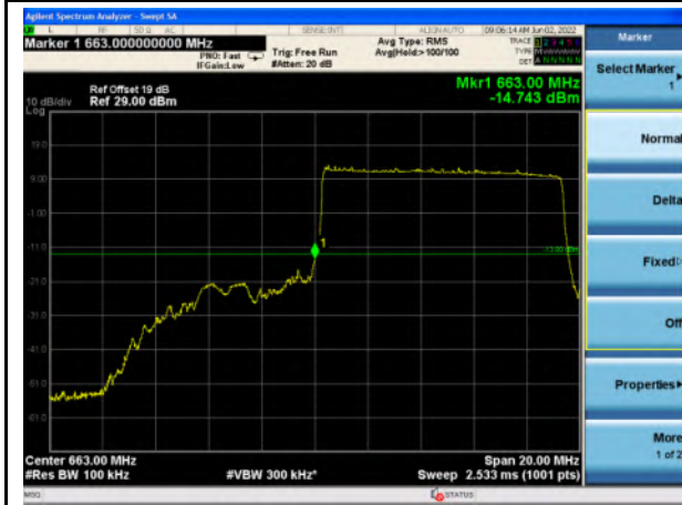
n71_10MHz_Lower Band Edge
