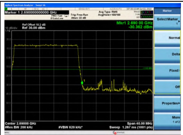
n41_20MHz_Upper Band Edge
