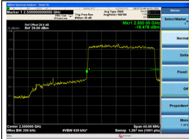
n7_20MHz_Lower Band Edge
