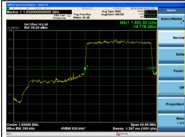
n2_20MHz_Lower Band Edge
