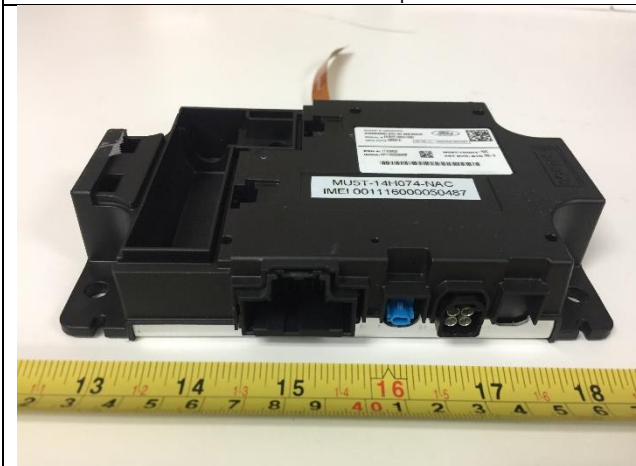
EUT-External-Front
