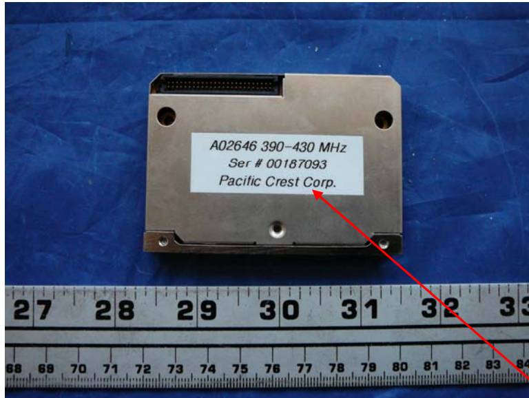
390~430 MHz
