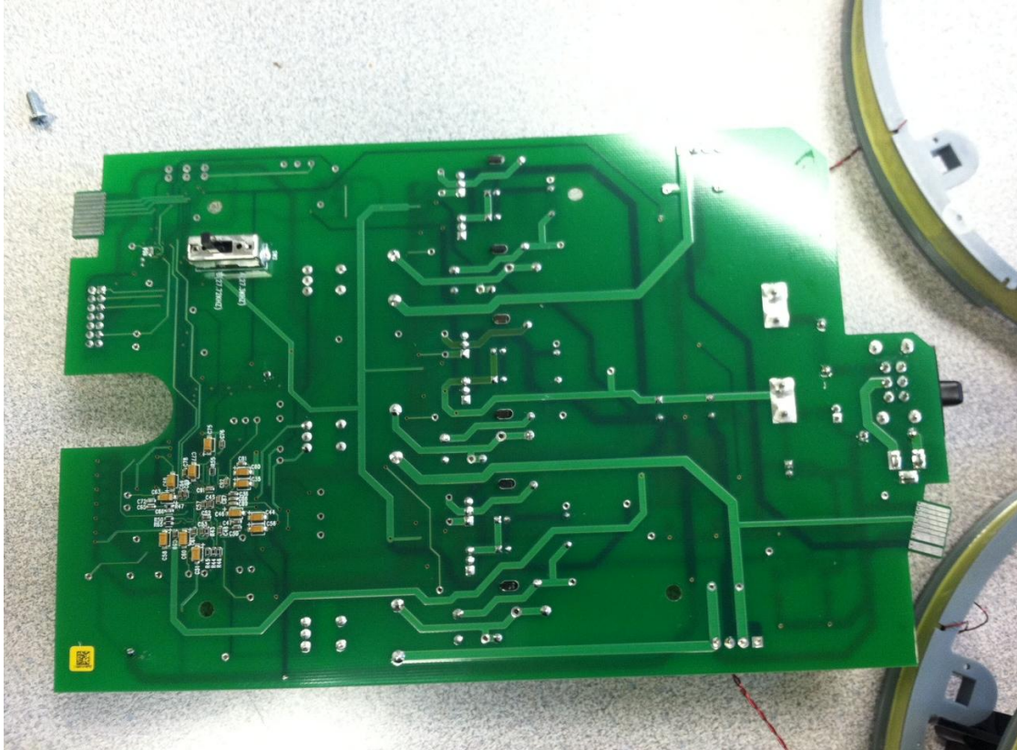
EUT PCB, Back Side
